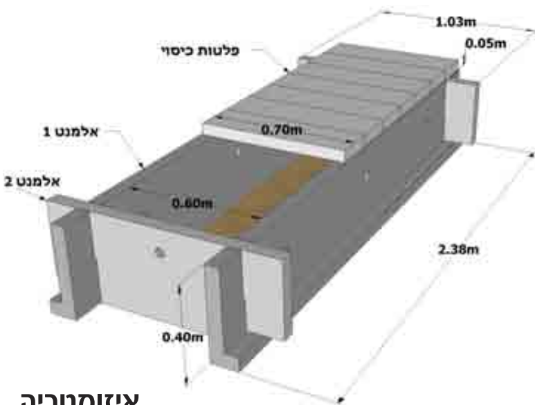
איזומטריה
